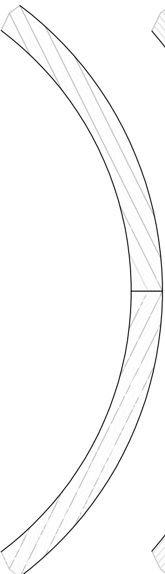
Bogen aus geraden Lamellen verleimt und im Bogen gefräst
